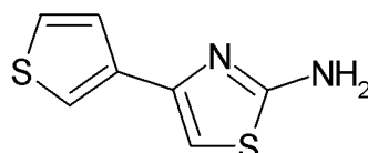
4-thien-3-yl-1,3-thiazol-2-amine KTD-502
